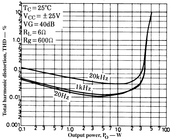
THD — P_O
